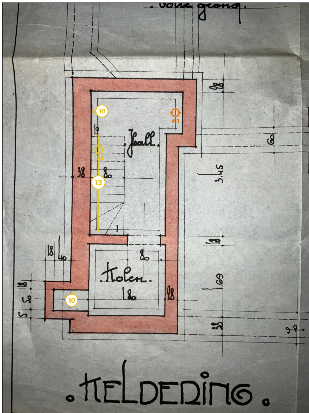
Legende van plan 1.1: -1 kelder
